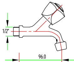
902 02HS WF-260 ก๊อกคอลันเซรามิคควาล์วหัวสามเหลี่ยม
