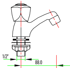
902 02VS BF-240 ก๊อกอ่างล้างหน้าเซรามิคควาล์วหัวสามเหลี่ยม
