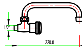
902 02HS SF-55C ก๊อกซิงค์ติดกำแพงเซรามิคควาล์ว แบบ C
