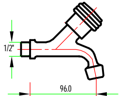
902 02HS WF-241 ก๊อกคอลันเซรามิคควาล์ว
