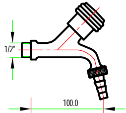
902 02HS WF-242 ก๊อกสนามเซรามิคควาล์ว 1/2"
