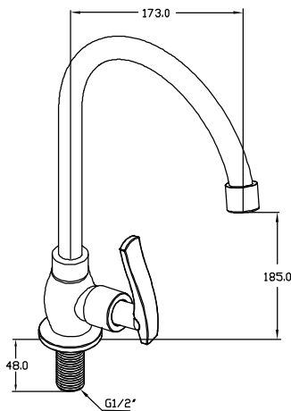
ก๊อกซิงค์ติดตั้งเคาน์เตอร์เซรามิกควาล์ว SF-119J (ปริมาณน้ำสูงสุดไม่เกิน 6 ลิตร/นาที่/1 bar)
