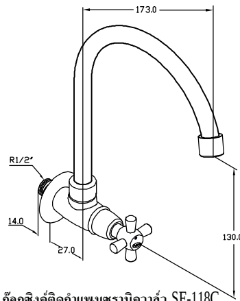
ก๊อกซิงค์ติดกำแพงเซรามิกควาล์ว SF-118C (ปริมาณน้ำสูงสุดไม่เกิน 6 ลิตร/นาที/1bar)
