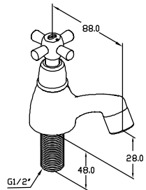
ก๊อกอ่างล้างหน้าเซรามิกควาล์ว BF-118 (ปริมาณน้ำสูงสุดไม่เกิน 6 ลิตร/นาที/1bar)
