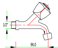
902 02HS WF-260 ก๊อกคอส์เซรามิคควาล์วหัวสามเหลี่ยม
