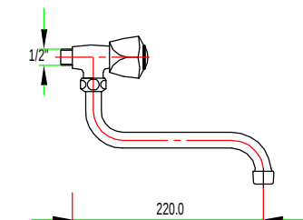
902 02VS SF-105S ก๊อกซิงค์เซรามิคควาล์วแป๊ป S หัวสามเหลี่ยม
