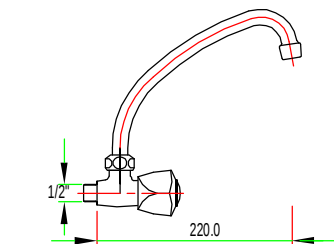
902 02VS SF-105C ก๊อกซิงค์เซรามิคควาล์วแป๊ป C หัวสามเหลี่ยม
