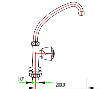
902 02VS SF-103J ก๊อกซิงค์เซรามิคควาล์วแป๊ป J หัวสามเหลี่ยม
