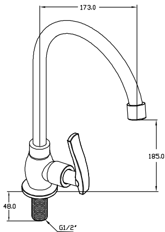
ก๊อกซิงค์ตั้งเคาน์เตอร์เซรามิกควาล์ว SF-119J (ปริมาณน้ำสูงสุดไม่เกิน 6 ลิตร/นาที่/1 bar)
