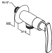
ก๊อกฝักบัวเซรามิกควาล์ว WF-119
