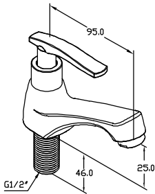
ก๊อกอ่างล้างหน้าเซรามิกควาล์ว BF-119 (ปริมาณน้ำสูงสุดไม่เกิน 6 ลิตร/นาที่/1 bar)
